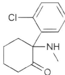
Ketamine
