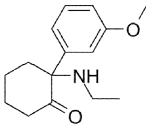
Methoxetamine (MXE)
